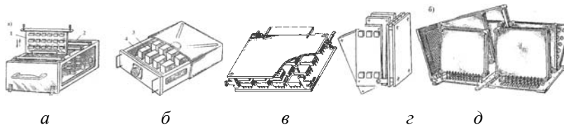
Рис. 3. Компонівка блоків: а) гребінчаста; б) пласка в) касетна, складена з двох плат; з) віялова; д) книжкова
