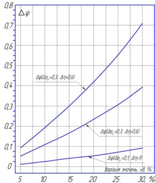
Рис. 1. Залежність використаного ресурсу пластичності \Delta\psi від величини варіації значень кривої граничних деформацій
