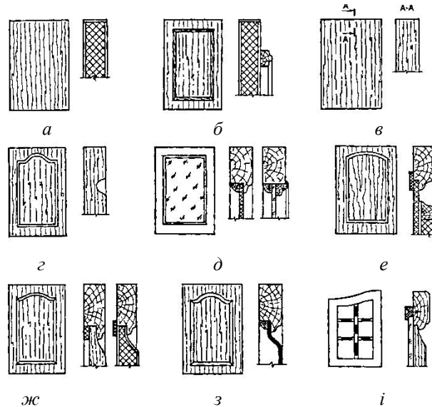
Рис. 1. Різновиди конструкції фасадів корпусних меблевих виробів: а) щитова з облицьованої плити; б) щитова з облицьованої плити з накладним декором; в) щитова з масивної деревини; г) щитова з масивної деревини з декоративною профільною обробкою лицевої площини; д) рамкова з тахлею з облицьованої фанери; е) рамкова з облицьованою тахлею і накладним декоративним щитком; ж) рамкова з тахлею з масивної деревини; з) рамкова з тонкою 3–4 мм формованою тахлею із шпону; і) рамкова засклена з накладною дерев'яною решіткою
