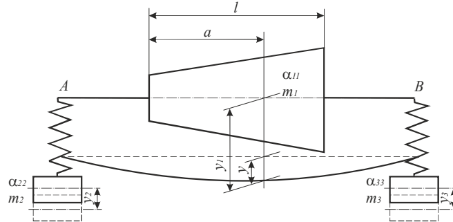
Рис. 1. Динамічна модель для розрахунку спільних коливань ротор-опори
