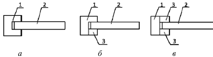
Рис. 3. Схематичне зображення конструкції кріплення тахлі рамкових фасадів: а ) в шпунт; б ) в фальц; в ) розкладками двосторонніми: 1 – брусок рамки; 2 – тахля; 3 – розкладки (штапики)
