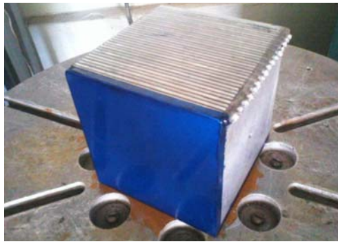
Рис. 3. Електростатичний кріпильний пристрій з нанесеною паяльною маскою
