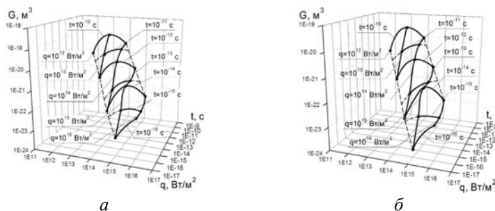
Рис. 3. Зависимость объема нанокластера от плотности теплового потока лазерного излучения q и времени его действия t в зоне, где образуются наноструктуры при R=10^{-6} м (а) и R=5 \cdot 10^{-7} м (б) для Т5К10
