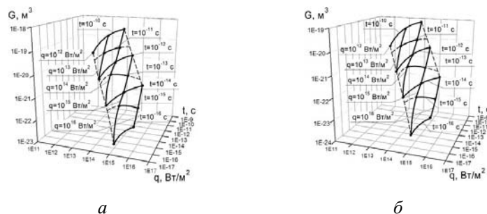
Рис. 2. Зависимость объема нанокластера от плотности теплового потока лазерного излучения q и времени его действия t в зоне, где образуются наноструктуры при R=10^{-6} м (а) и R=5 \cdot 10^{-7} м (б) для ВК4
