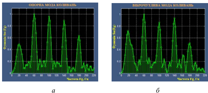
Рис. 2. Спектральне представлення реакції КР в умовах зовнішніх комплексних вібромеханічних впливів для частот 20 Гц, 60 Гц, 100 Гц, 140 Гц і 180 Гц для основної (а) та третьої (б) гармонік
