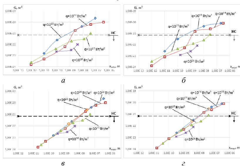
Рис. 1. Зависимость объёма нанокластера от минимальной (а, б) и максимальной глубины (в, г) при действии лазерного излучения с различной плотностью теплового потока q , материал Р9 (а, в) и Т30К4 (б, г) R_n = 5 \cdot 10^{-7} м
