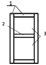
Рис. 2 – Конструкція фасаду: 1 – обв'язка; 2 – середник; 3 – фільонки
