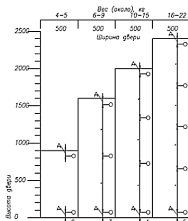
Рис. 5. Рекомендований присадний ряд встановлення завіс на один фасад
