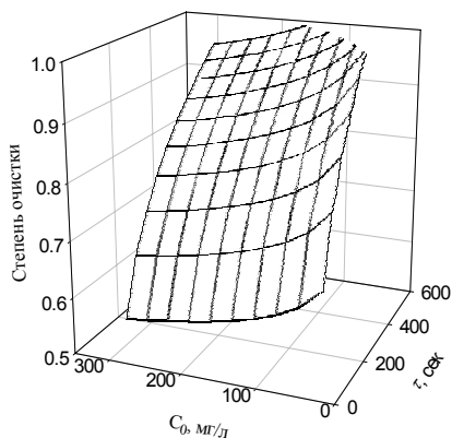
Рис. 1. Зависимость степени очистки раствора от начальной концентрации ПАОВ и времени обработки
