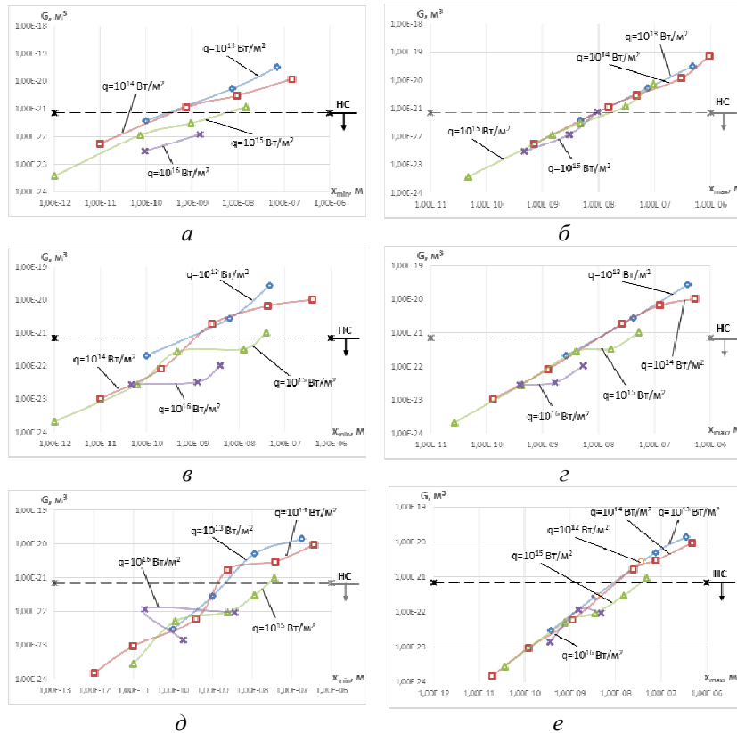
Рис. 1. Зависимость объёма нанокластера от минимальной (а, в, д) и максимальной (б, г, е) при действии лазерного излучения с различной плотностью теплового потока q при R = 5 \cdot 10^{-7} м для ВК4 (а, д), Т5К10 (в, г) и ТТ20К9 (д, е)
