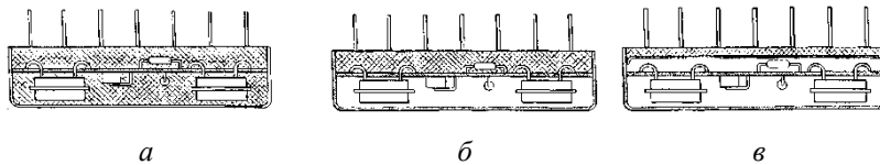
Рис. 2. Мікромодулі різних конструкцій: а) монтажна; б) напівпустотіла; в) пустотіла
