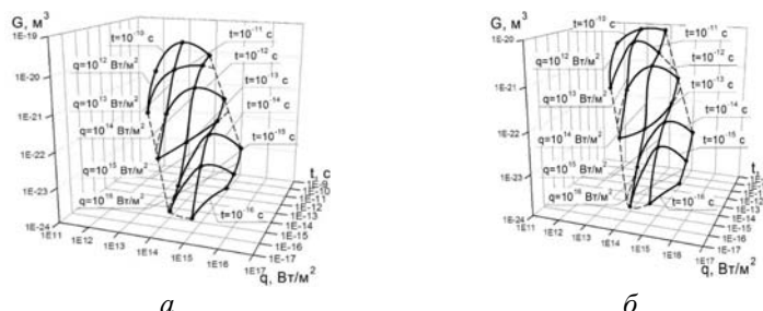
Рис. 2. Зависимость объёма нанокластера от плотности теплового потока лазерного излучения q и времени его действия t в зоне, где образуются наноструктуры R_n = 5 \cdot 10^{-7} м для БС Р9 (а) и ТС ТЗ0К4 (б)
